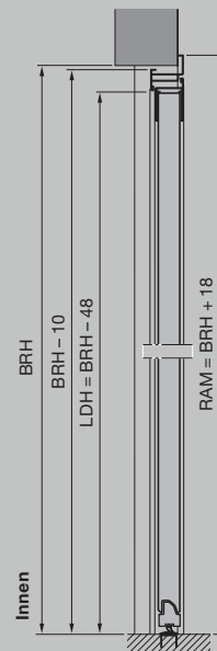
Nebentür mit Alu-Eckzarge Profiltyp 2 Außenschlag
