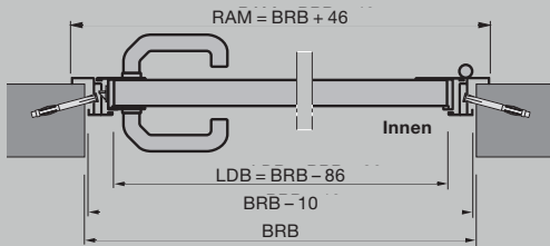
Nebentür mit Alu-Eckzarge Profiltyp 3 Außenschlag
